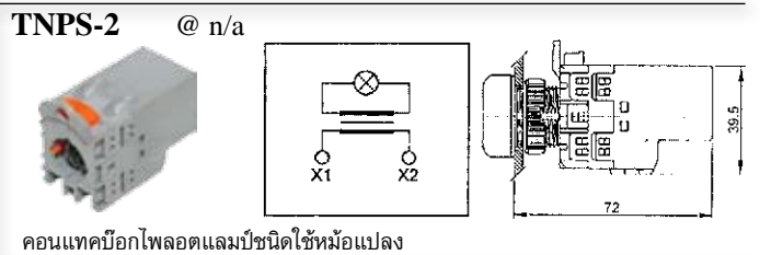
โพลอตแลมป์ชนิดใช้หม้อแปลง 30 มม.
